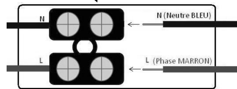
CONNEXIONS ELECTRIQUES
